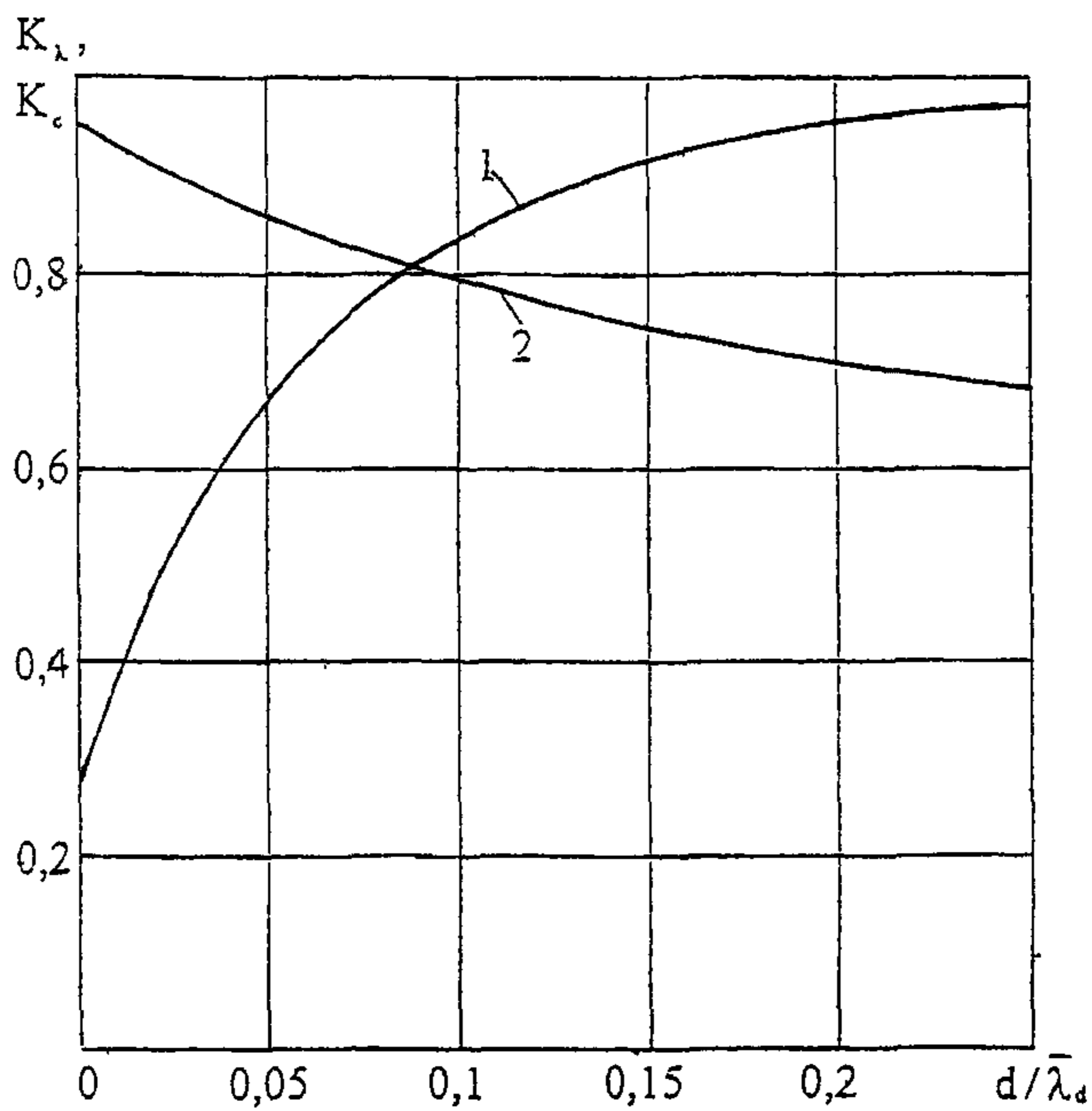
Рисунок А.2 - Графики для определения коэффициентов K_\lambda (1) и K_e (2)
