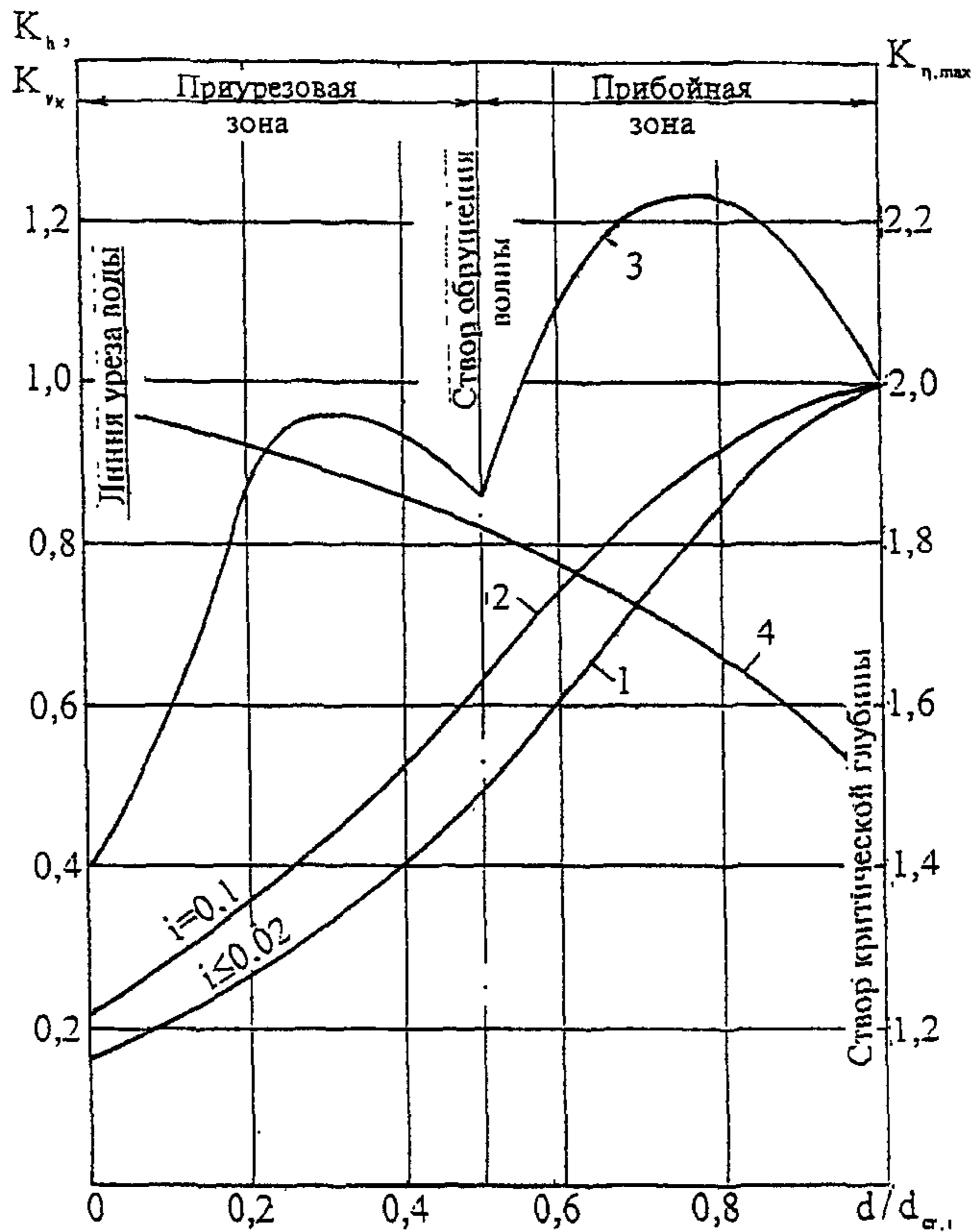
Рисунок А.3 - Графики для определения коэффициентов K_b (1 и 2), K_{vx} (3) и K_{\eta, max} (4)
