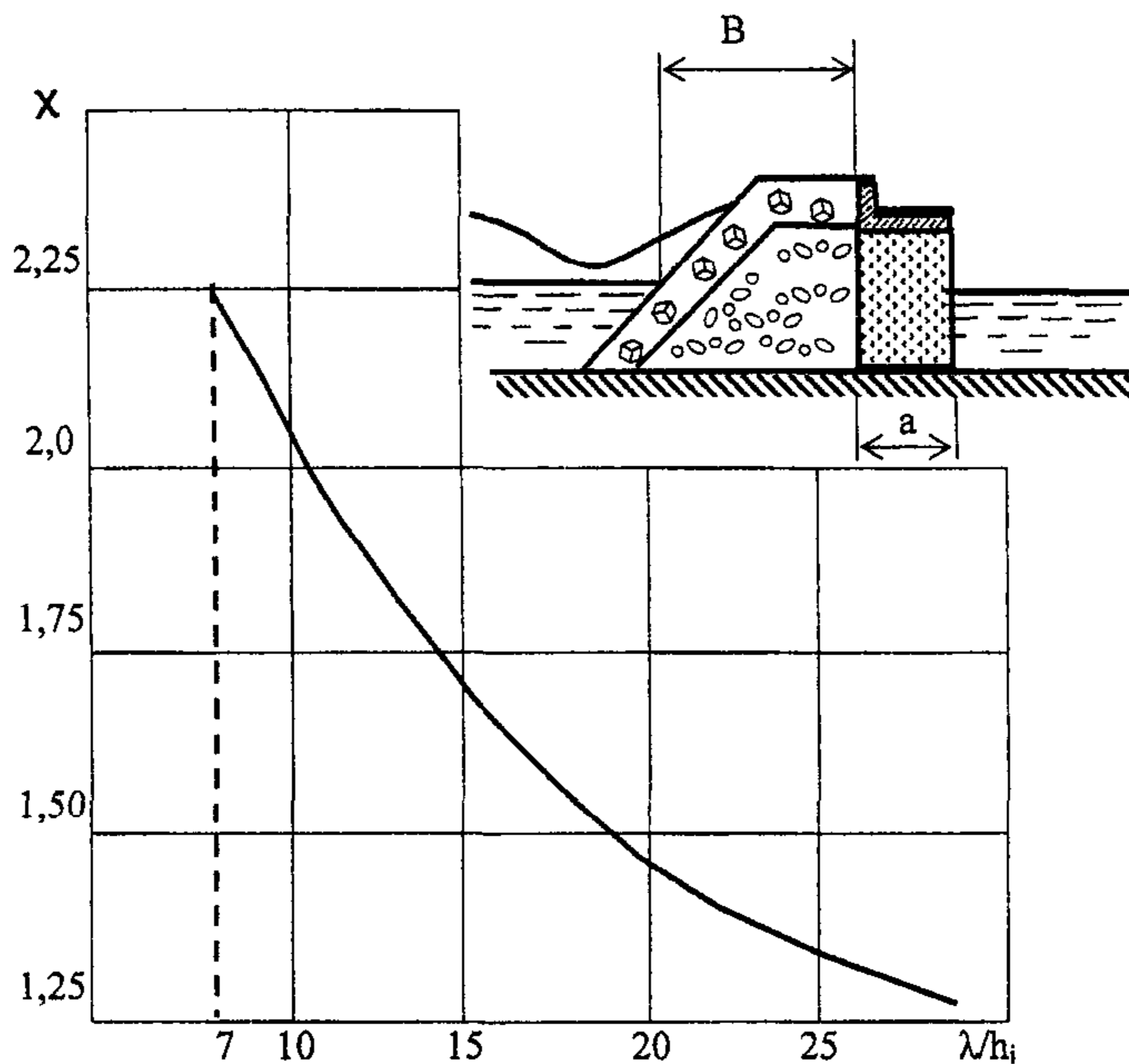
Рисунок 5.8 - График для определения коэффициента \chi = f(\bar{\lambda} / h)
