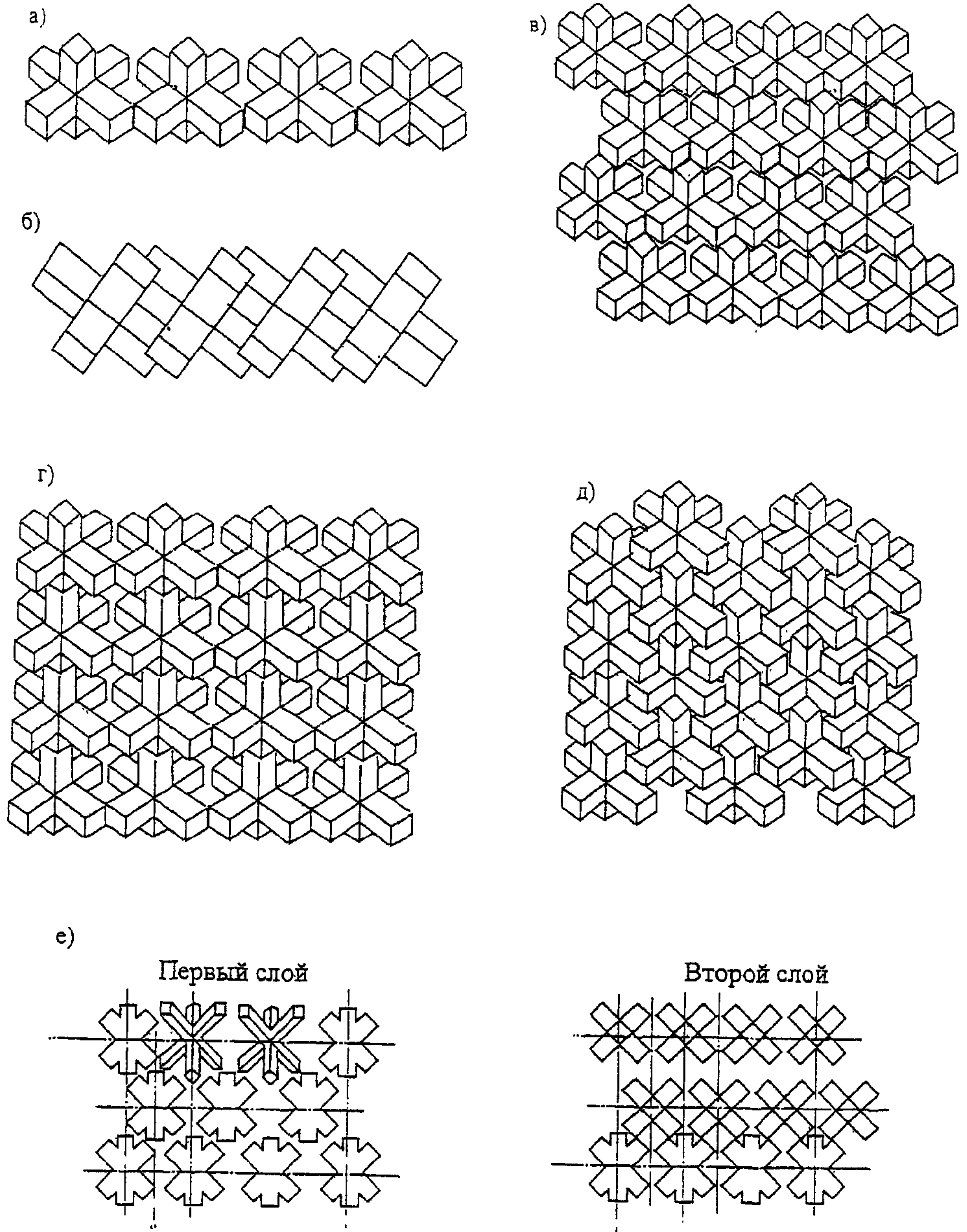
Рисунок Б.2 – Схемы укладки гексалегов на откосе
