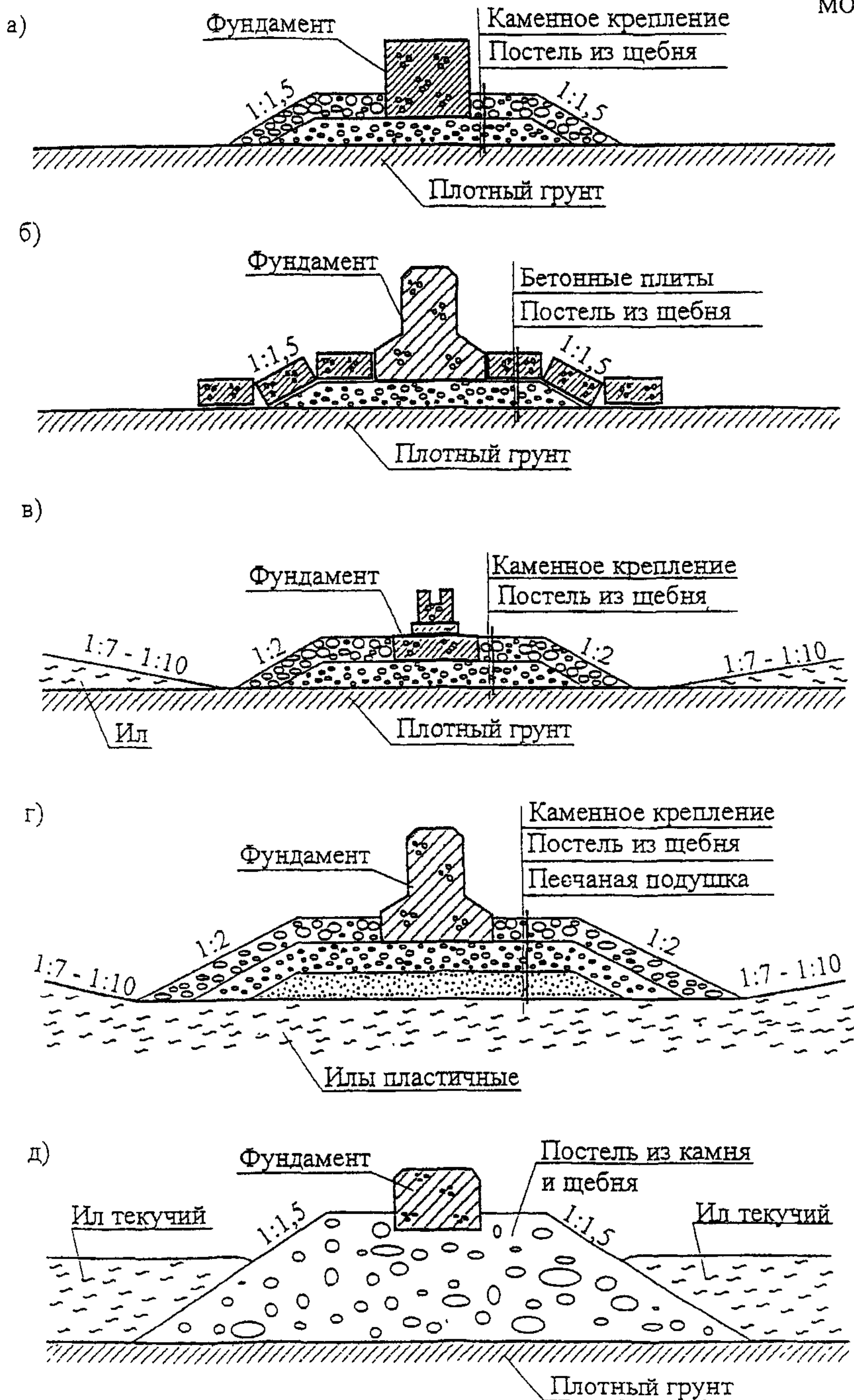
Рисунок 7.2 – Схемы конструкций подводных стендов
