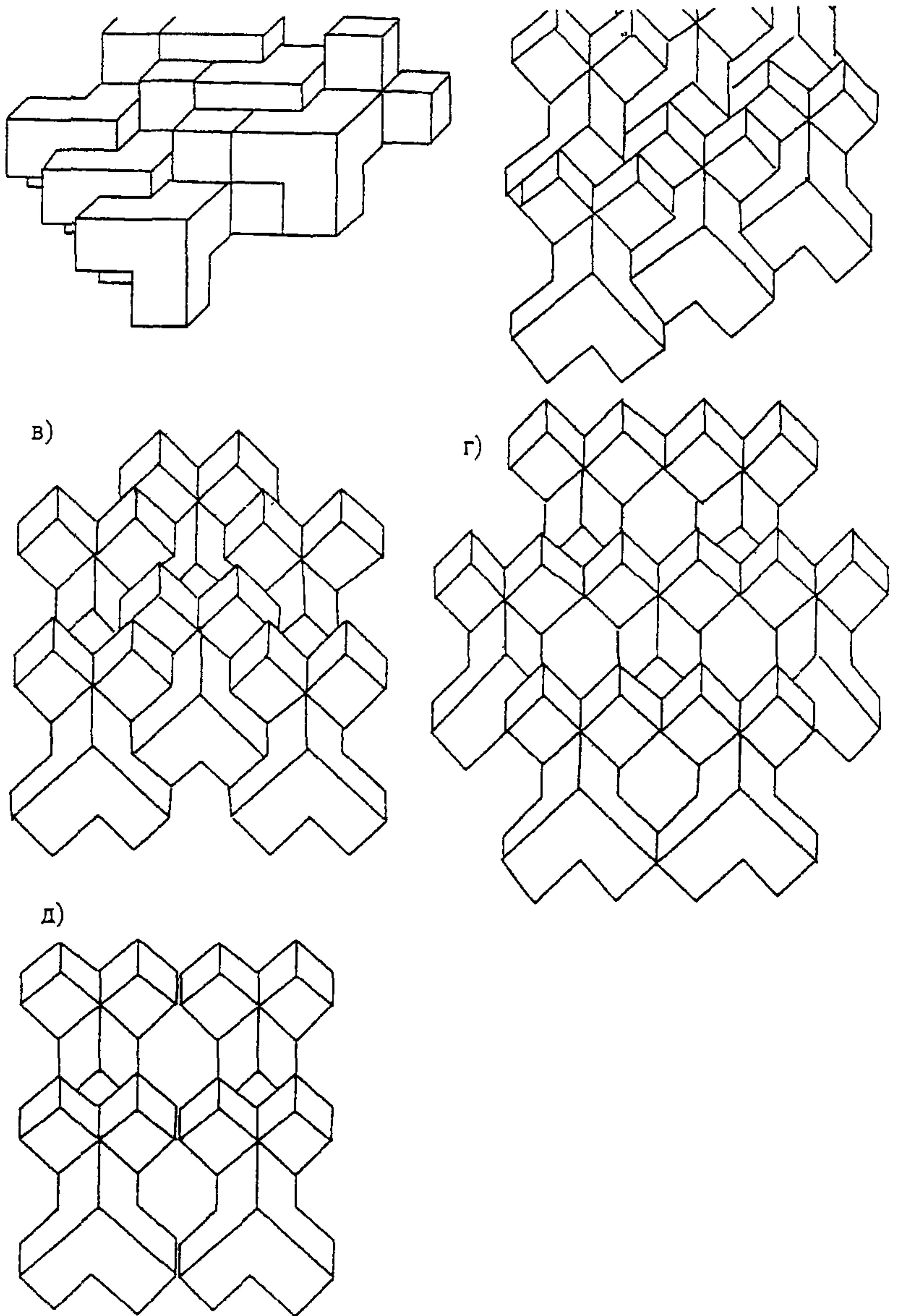
а – внахлест; б, в – с защемлением; г, д – встык Рисунок Б.4 – Схемы однослойной укладки пентаподов
